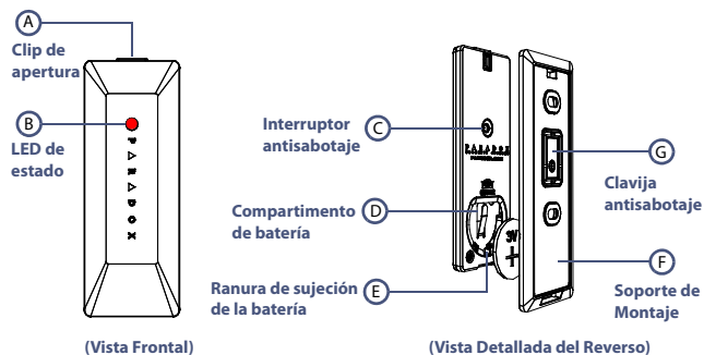
Figura 1: Vista del frente y reverso del GS250.
